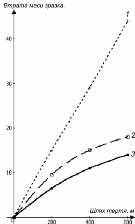
Рис. 1. Порівняльні показники зносу моносплаву бронзи і ЛКМ при зміні шляху тертя в умовах дії прошарку піску і постійного навантаження 4,5 кг: 1 – бронза; 2, 3 – ЛКМ (склади №604 і №900) відповідно
