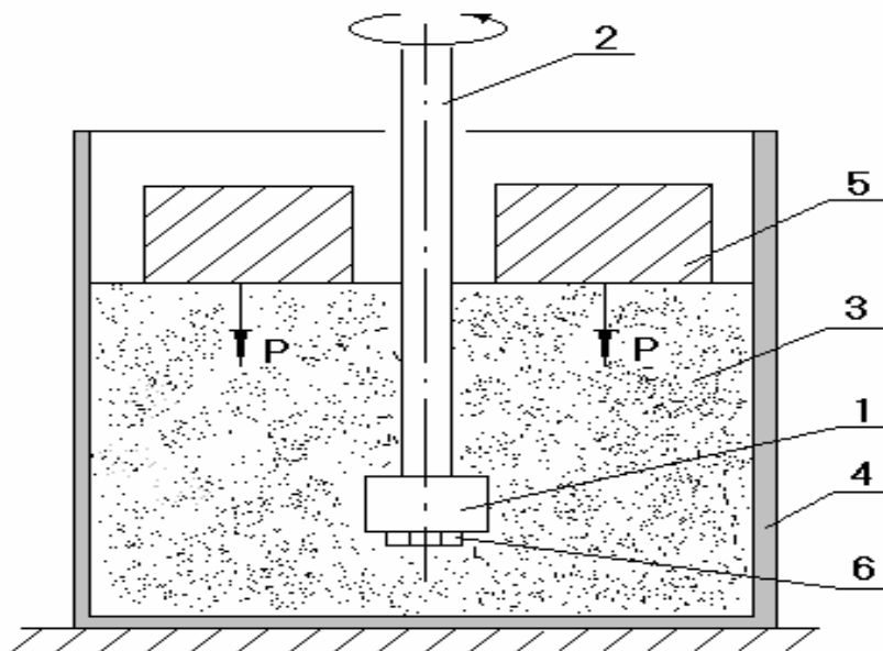
Рис. 2. Установка для дослідження абразивної зносостійкості ЛКМ і моносплавів, де: 1 – досліджуваний циліндричний зразок з отвором (моносплав або композит); 2 – вал; 3 – сипучий абразив; 4 – зовнішня поверхня установки («гільза»); 5 – навантажувальний диск з отвором; 6 – гвинт, що тримає досліджуваний зразок.
